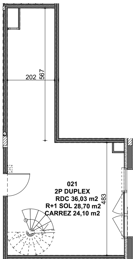
PLAN RDC
