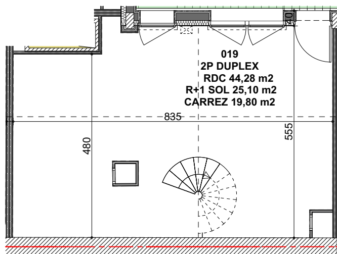
PLAN RDC
