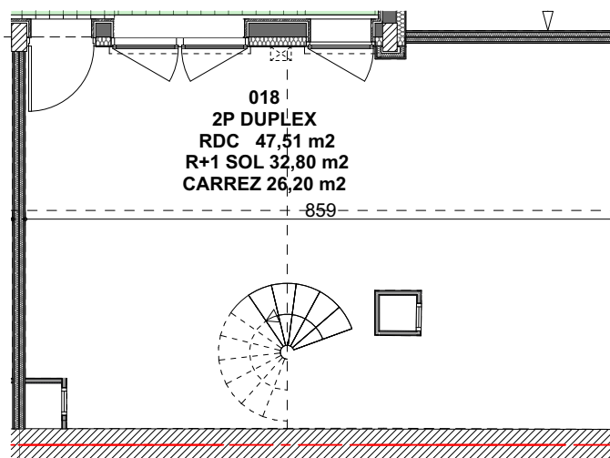
PLAN RDC
