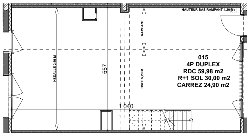
PLAN RDC
